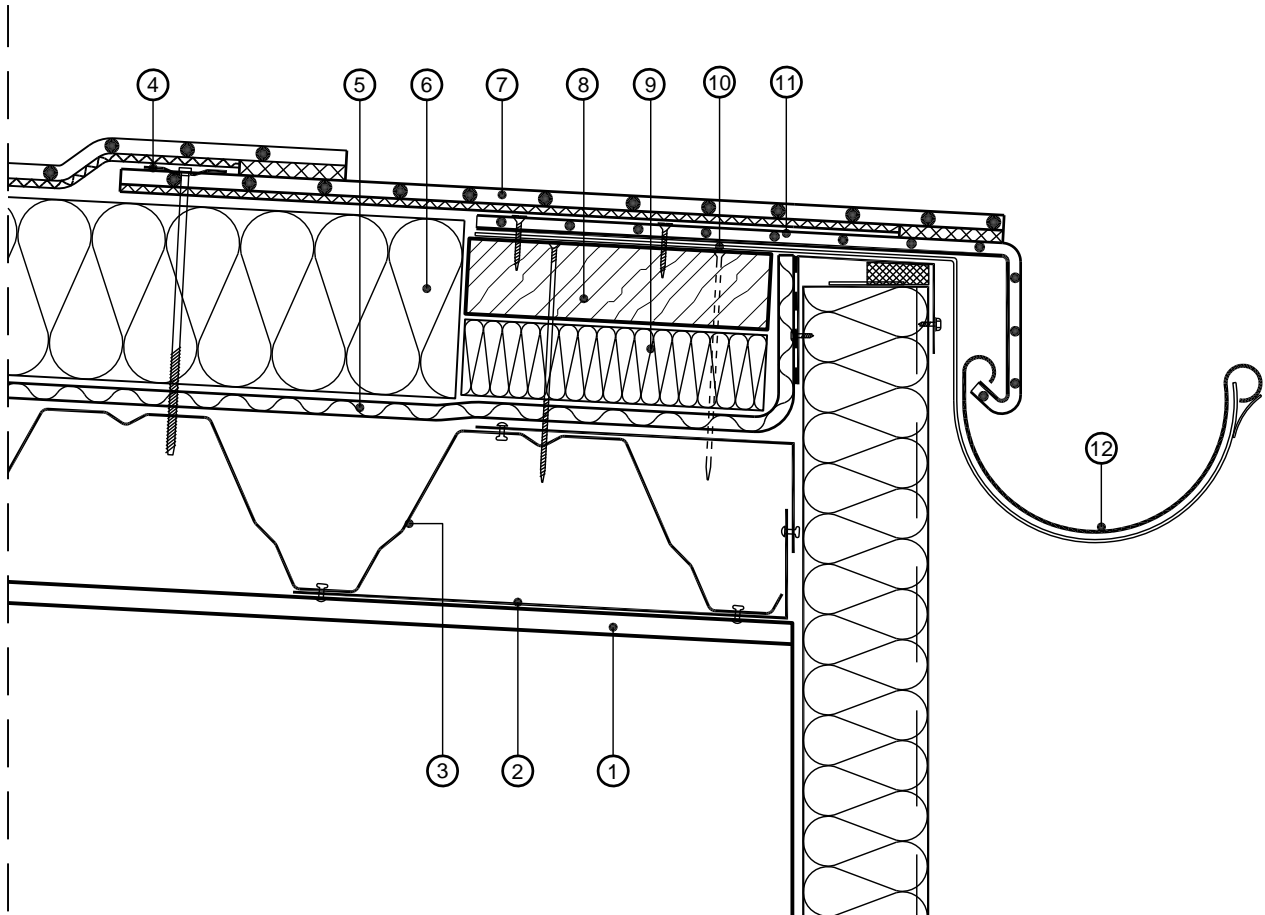
Maßstab 1 : 5 (Die für die Abdichtung relevanten Schichten sind überhöht dargestellt)
