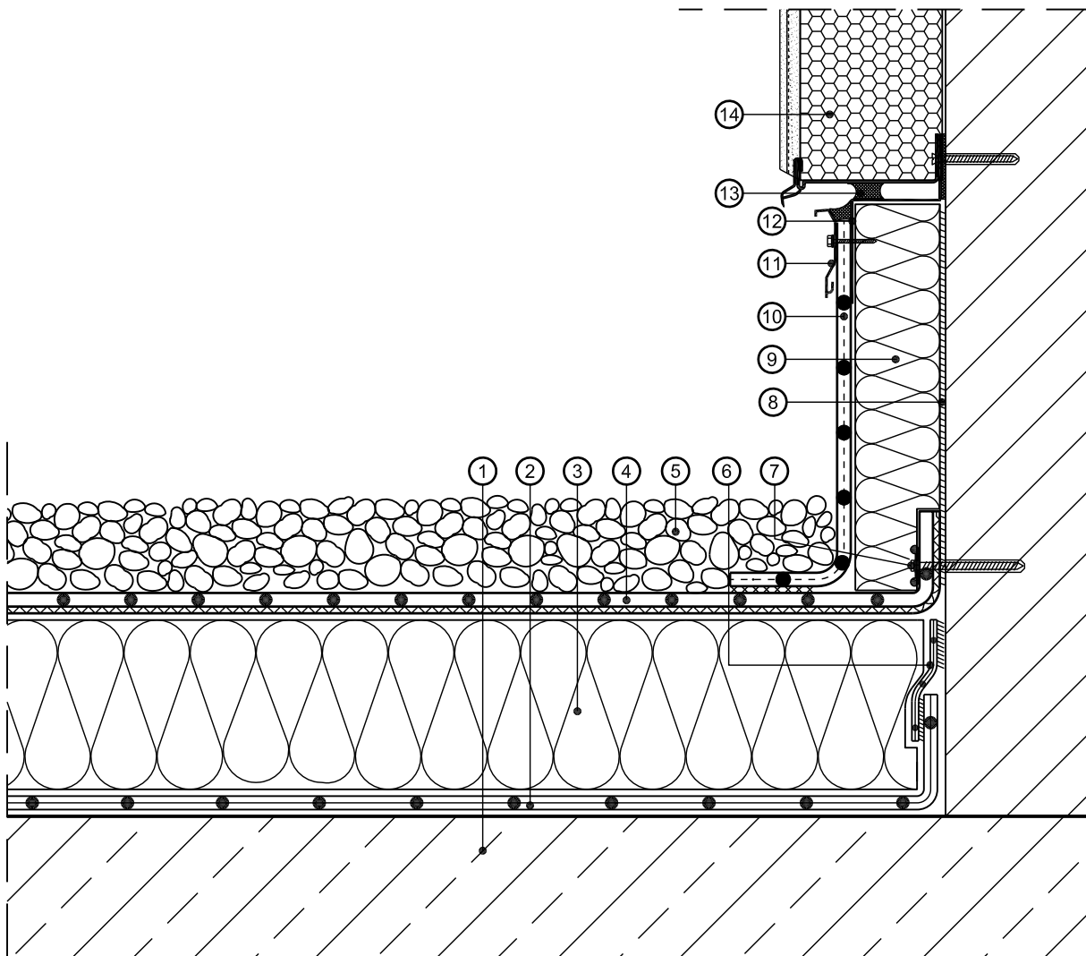
Maßstab 1 : 5 (Die für die Abdichtung relevanten Schichten sind überhöht dargestellt)
